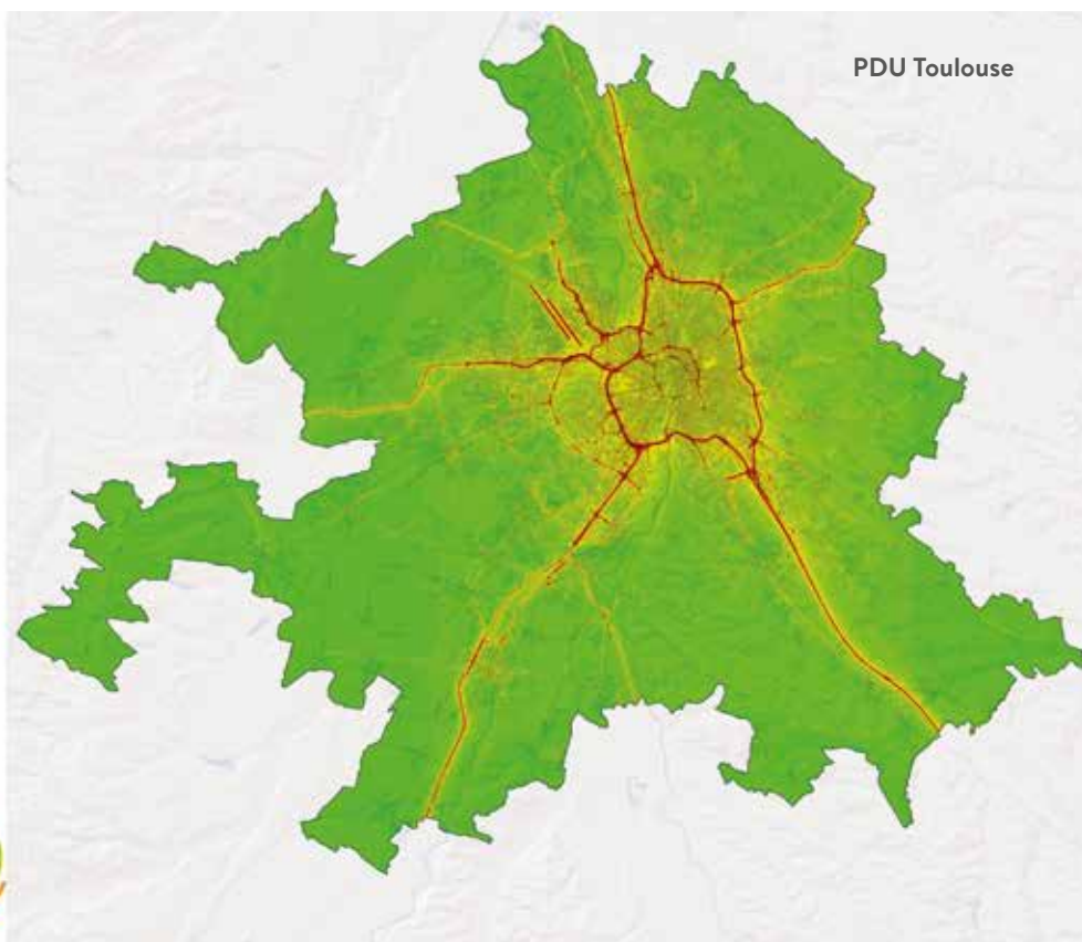
Situation des NO 2 pour la protection de la santé (en µg/m 3 - Moyenne annuelle)
