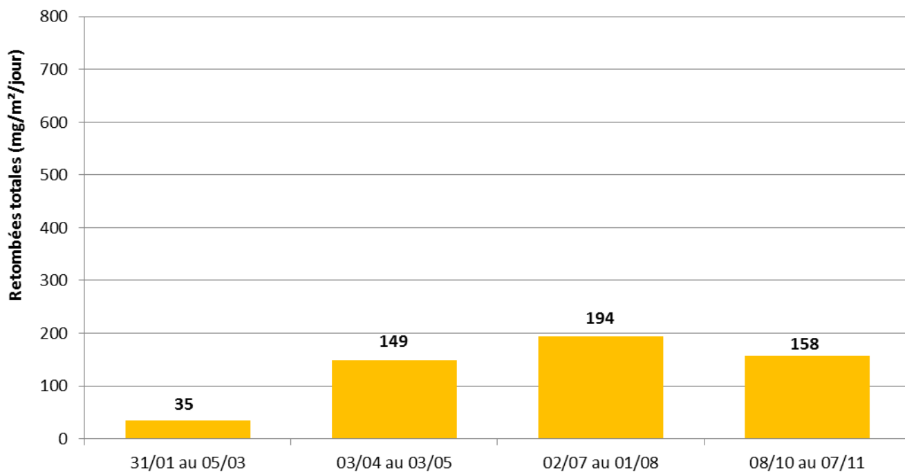
Suivi des retombées totales en 2019 – point de mesure RCI 4
