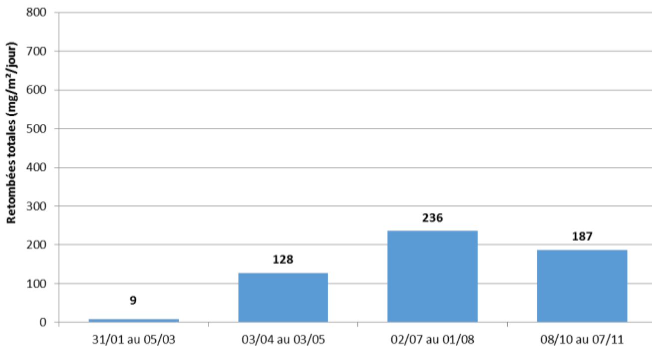
Suivi des retombées totales en 2019 – point de mesure RCI 4 (type a)
