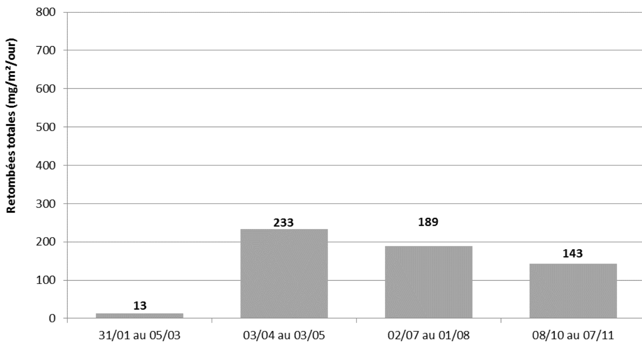
Suivi des retombées totales en 2019 – point de mesure RCI 3
