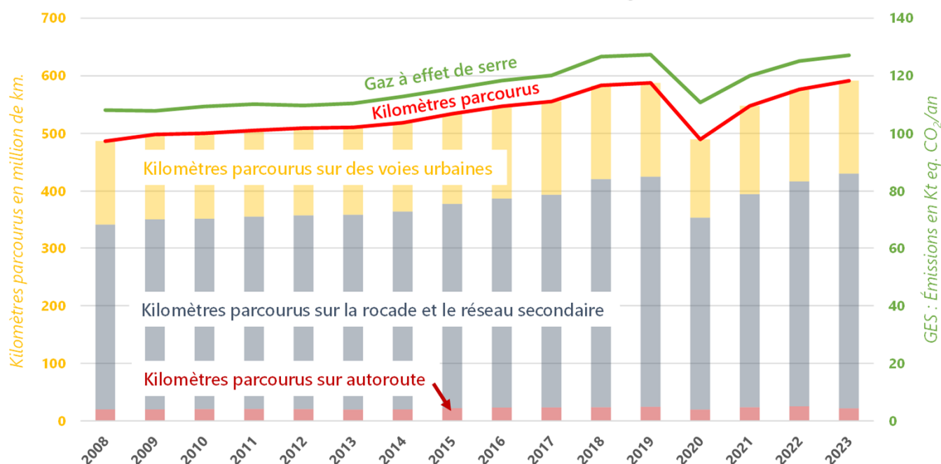
Évolution comparée des émissions de gaz à effet de serre et du trafic routier sur le territoire de l'Albigeois
